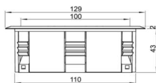
Einbauskitze in mm
