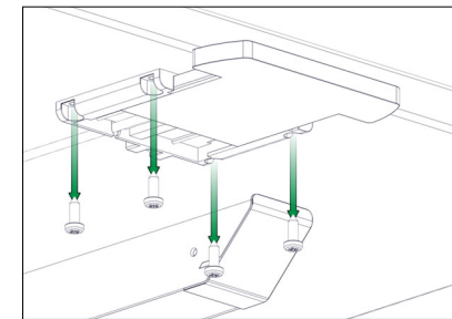
2 bedieningselement demonteren
