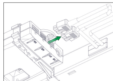
5 motorkabel uit de besturing verwijderen
